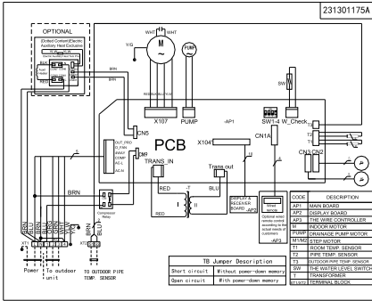
Схема для для внутренних блоков (модель LCAC-24TC)
