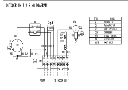
Схема для для наружных блоков (модель LCAC-24T)
