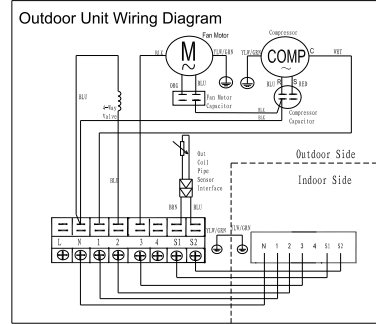
Схема для для наружных блоков (модель LCAC-12/18T)
