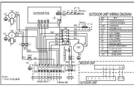
Схема для для наружных блоков (модель LCAC-48T)
