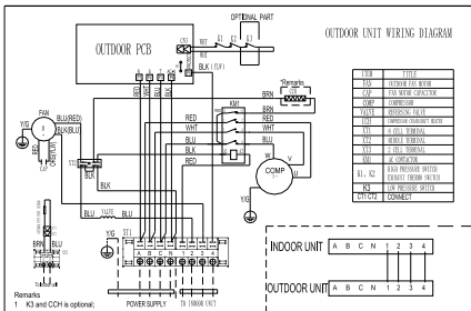
Схема для для наружных блоков (модель LCAC-36T)
